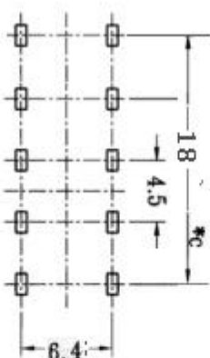
P.B.C LAYOUT
